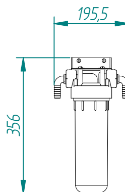
FILTRE D'ASPIRATION
