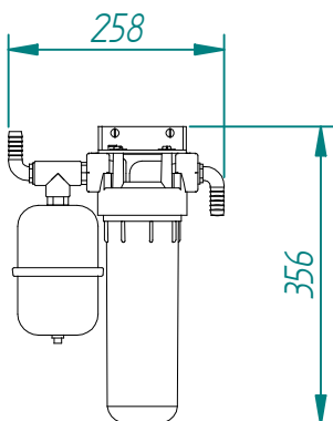
FILTRE 5 MICRONS
