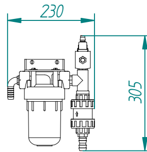
FILTRE D'ASPIRATION
