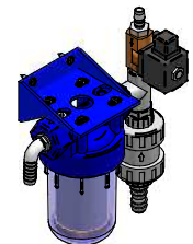
FILTRE D'ASPIRATION
