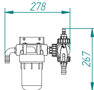
FILTRE D'ASPIRATION
