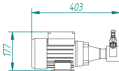
POMPE BASSE PRESSION 220 V AC
