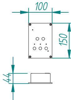
PANNEAU DE CONTRÔLE ELECTRONIQUE
